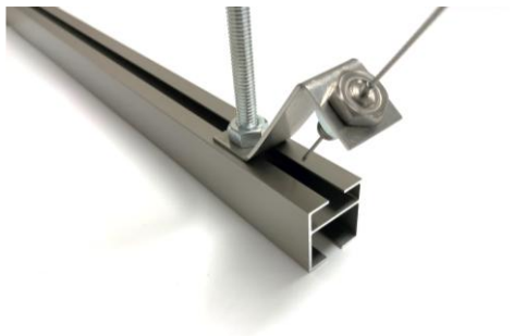
ワイヤー式振れ止め アルティマ ワイヤーロック(振れ止めワイヤーシステム) ※アルティマ ターンバックルを統合しております
