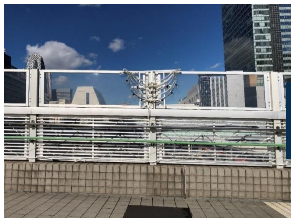
施工前_JR某駅南口ご線橋
